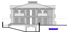
Elevation 02
